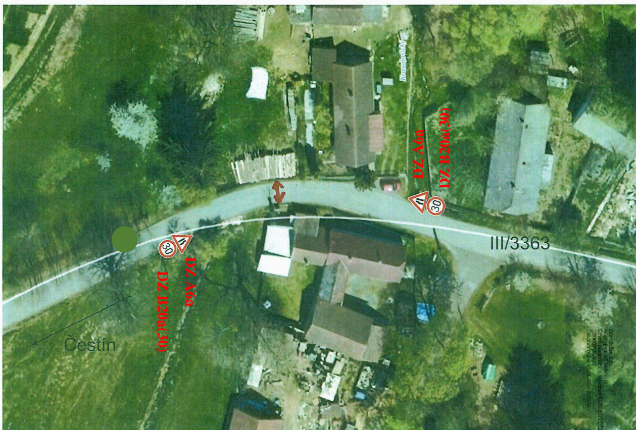
Sil. č. III/3363 v obci Krasoňovice, úprava provozu - zúžené místo
